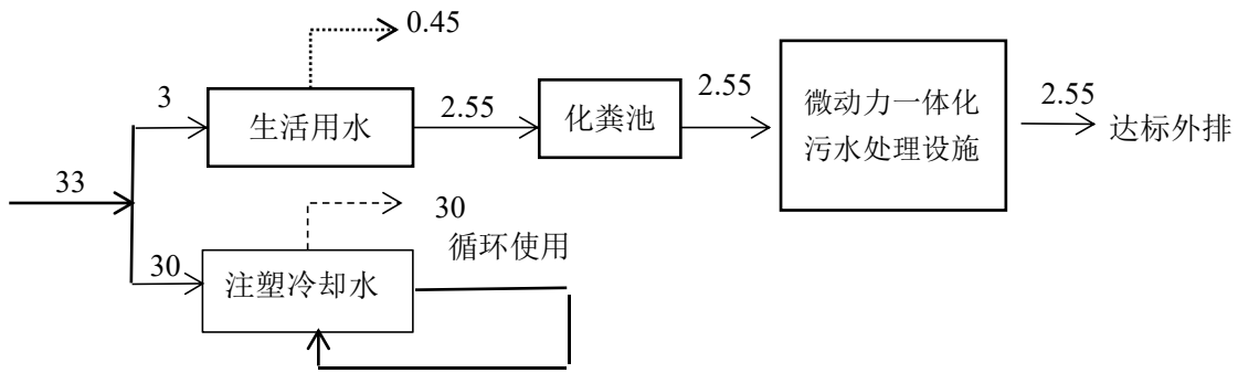
图 2-1 调试期间水平衡图 (单位 t)
