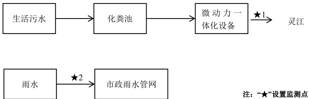
图3-1废水处理工艺流程图
