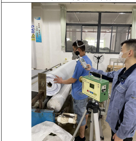
图 4 现场检测图
