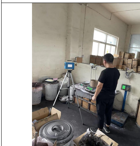
图 2 现场检测图
