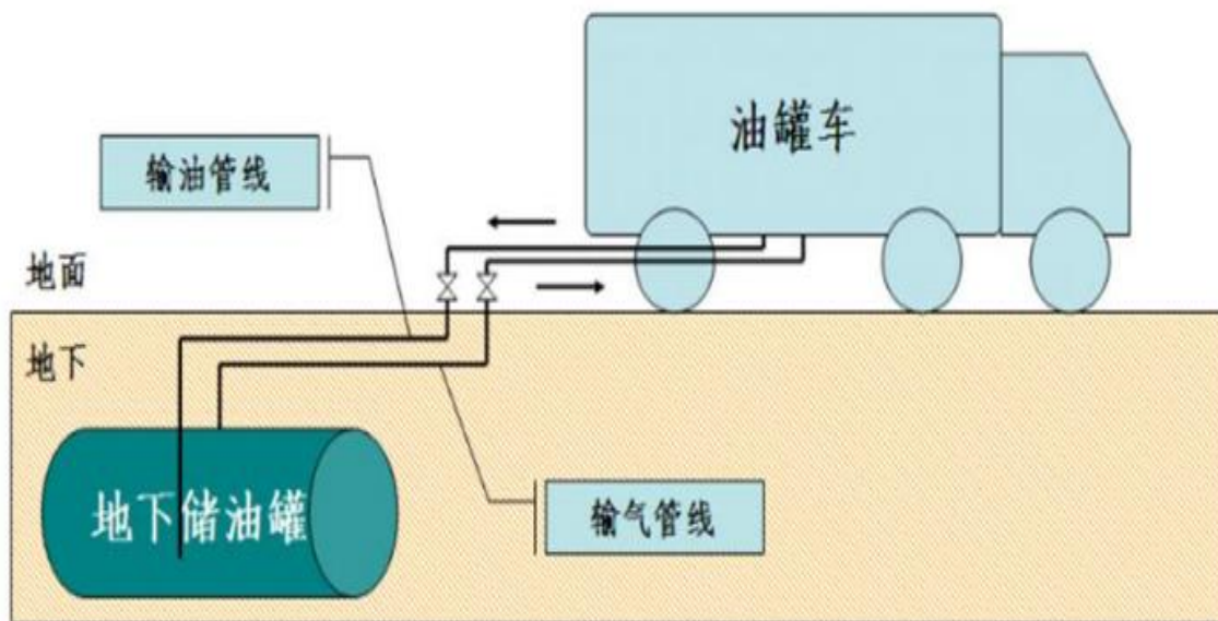
图 2-3 一次回收系统原理图
