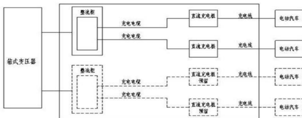
图 2-2 营运期电力销售流程图
