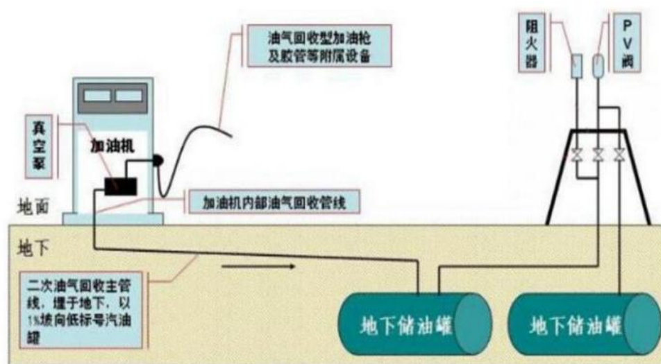
图 2-4 二次回收系统原理图
