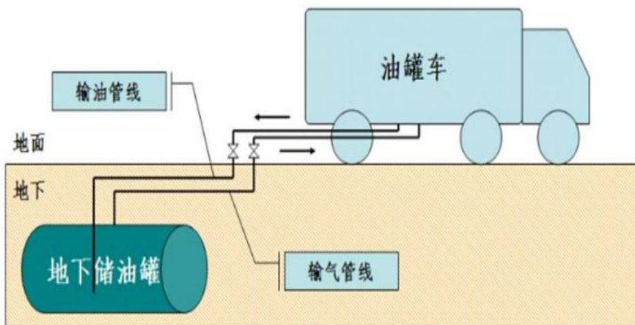
图 2-3 一次回收系统原理图
