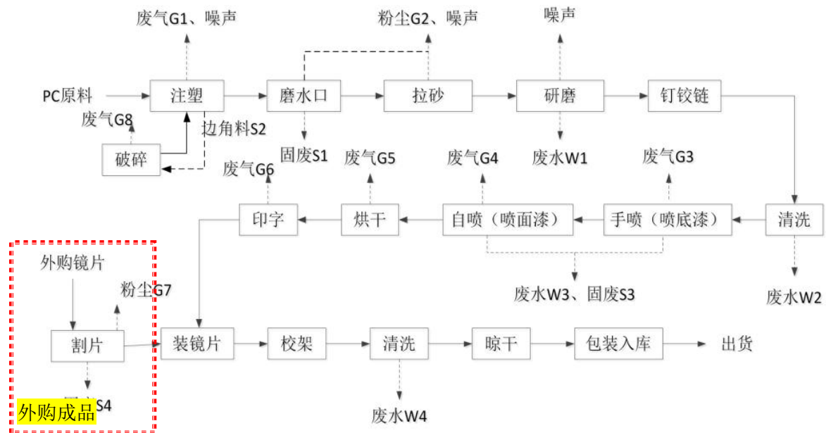
图 2-2 塑料眼镜生产工艺流程图
