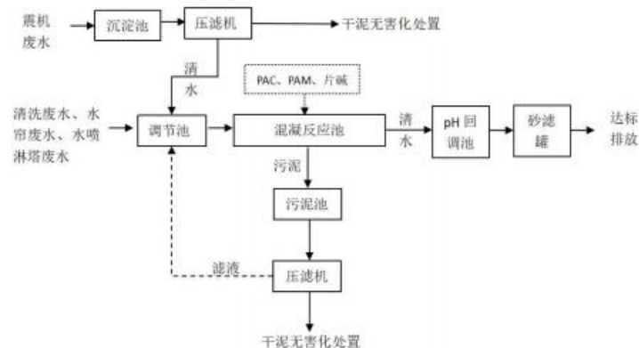
图 3-3 废水处理工艺流程图
