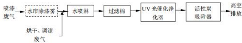
图 3-2 喷漆有机废气处理工艺原则流程图
