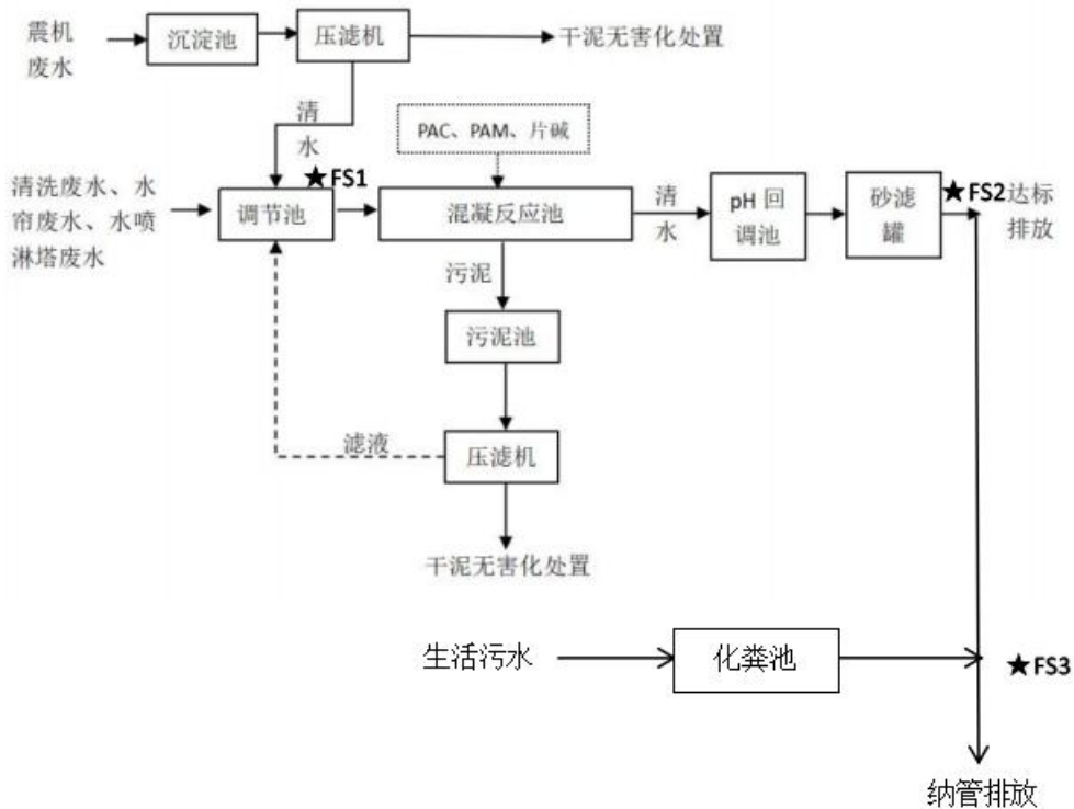
图 3-1 废水处理工艺
