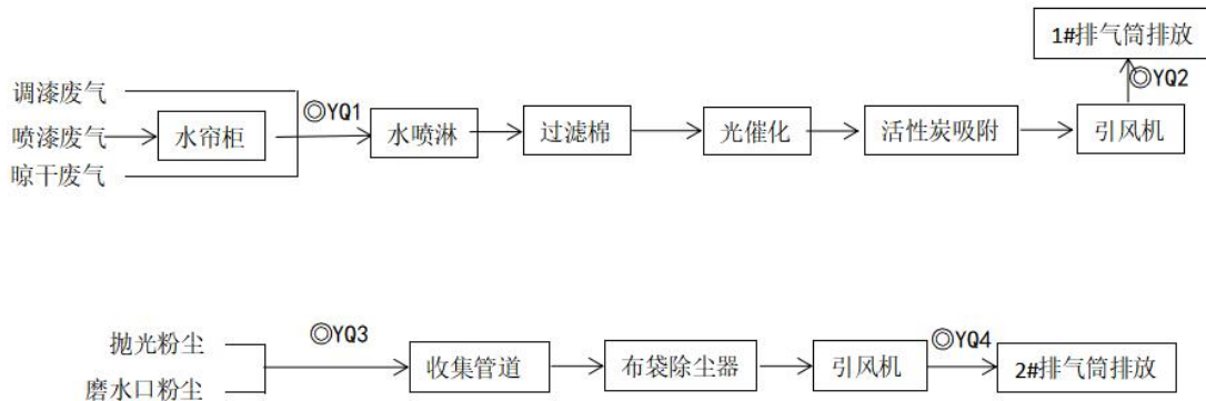
图 3-2 废气处理工艺
