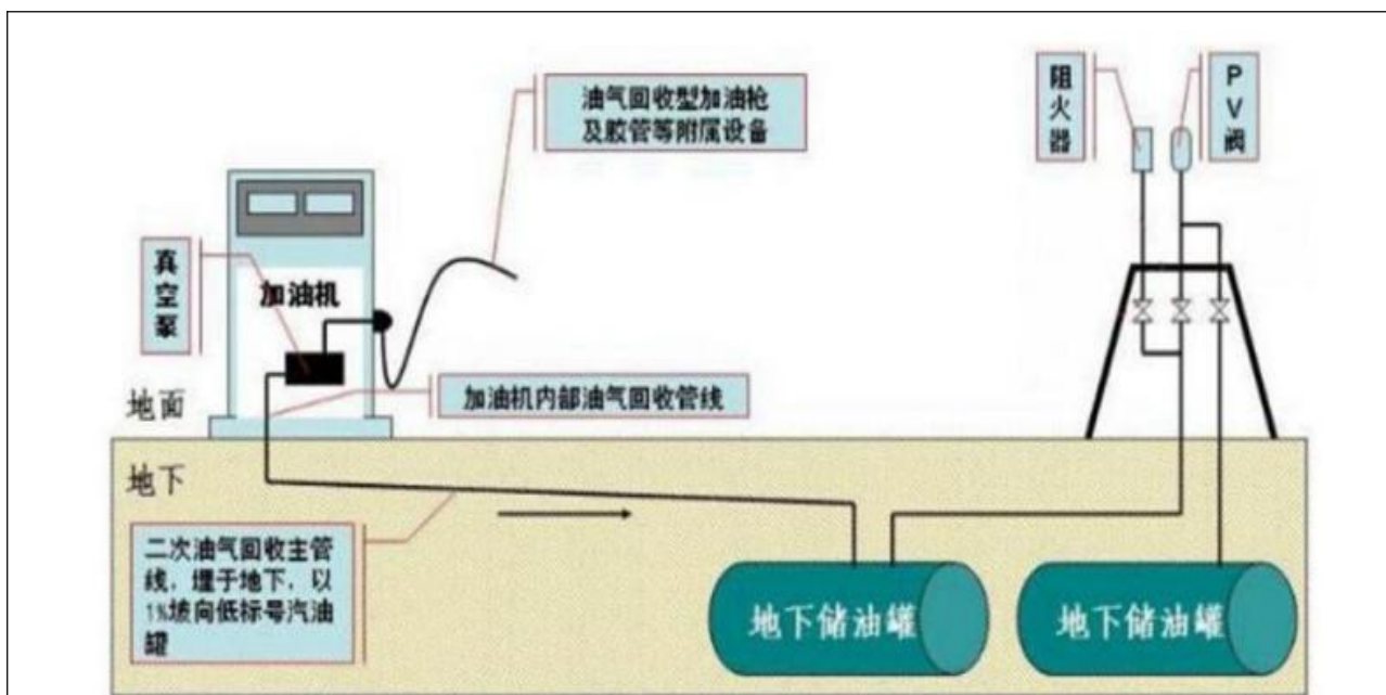
图 2-6 二次回收系统原理图
