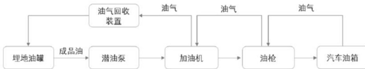
图 2-3 加油流程图
