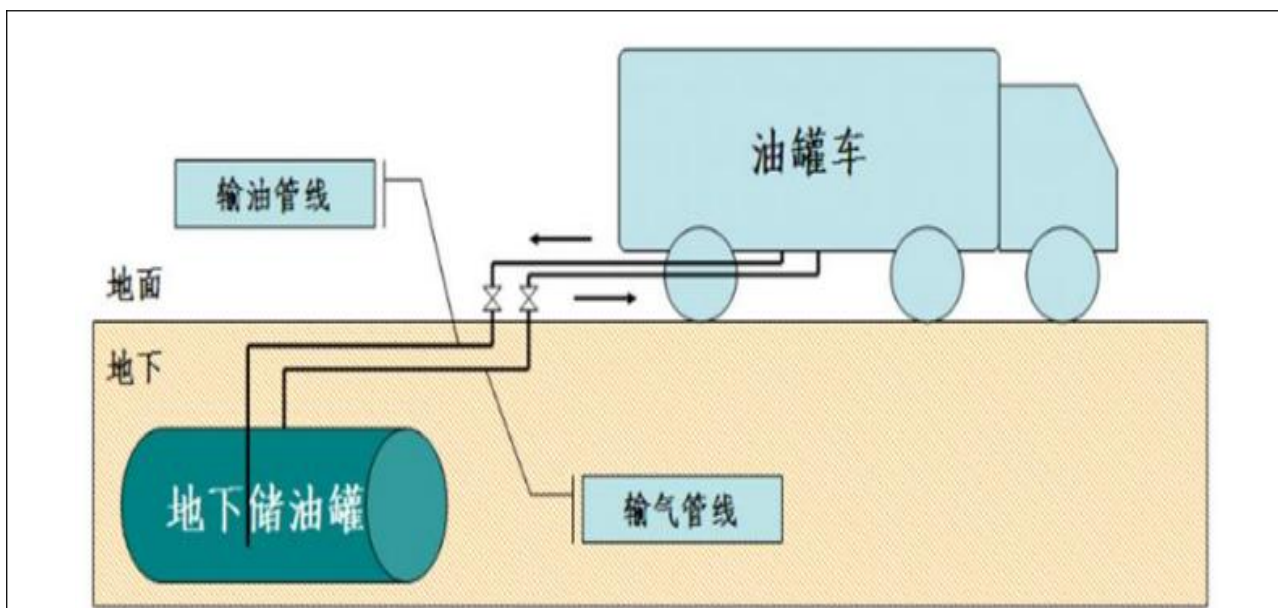
图 2-3 一次回收系统原理图
