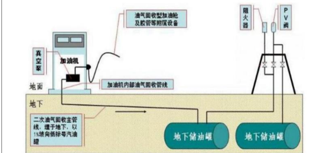
图 2-4 二次回收系统原理图
