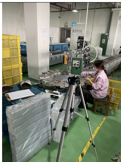
图 8 现场检测图
